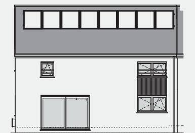
Pignon droit
